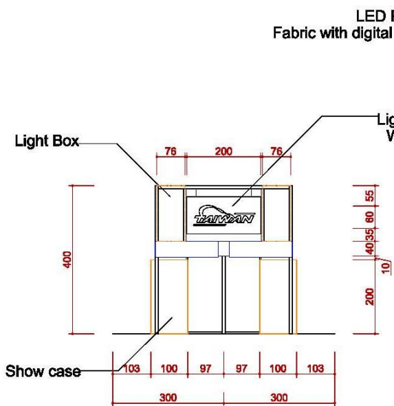
1 C-1 ELEVATION
